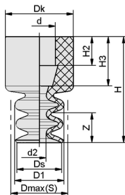
Données de construction FG 9 HT1-60 N016
