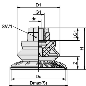
デザインデータ SAB 50 NBR-60 G1/4-IG
