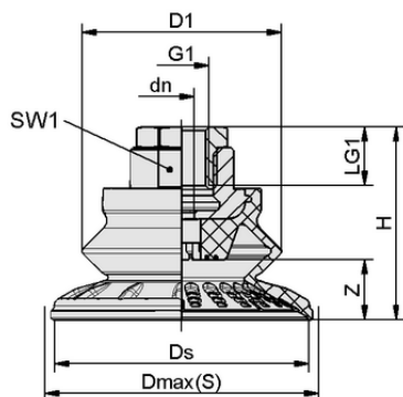
Конструктивные данные SAB 80 NBR-60 G1/4-IG
