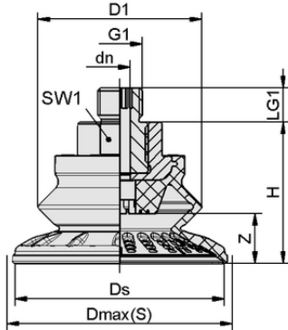
Tasarım verileri SAB 50 NBR-60 G1/4-AG
