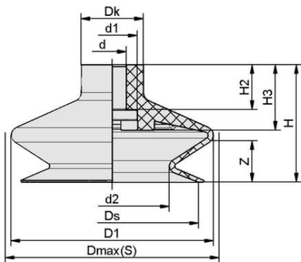
Datos de diseño FGA 63 SI-55 N018
