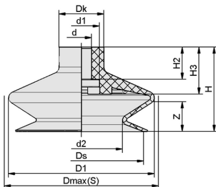
Dati di costruzione FGA 63 NBR-55 N018
