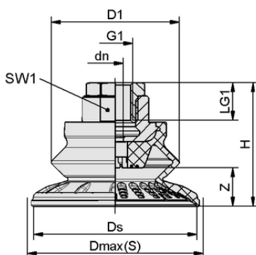
Données de construction SAB 100 NBR-60 G3/8-IG
