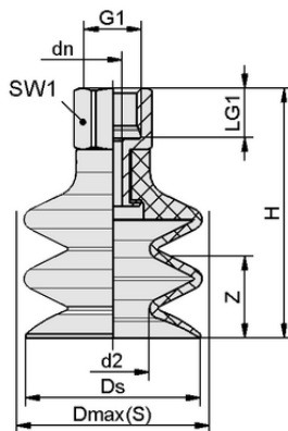
Design data FSG 5 SI-55 M5-IG
