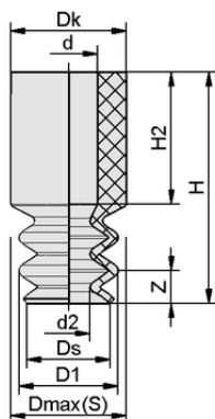
Datos de diseño FG 5 NBR-CO-55 N017
