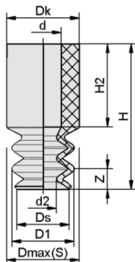
Конструктивные данные FG 5 NBR-55 N017
