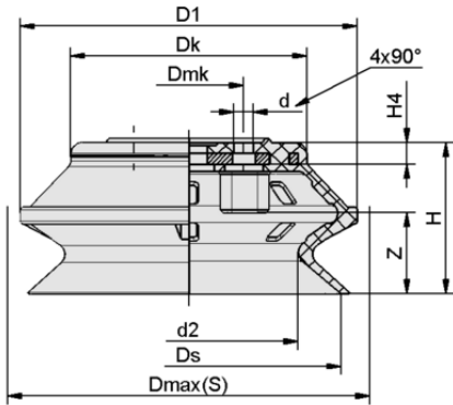
Tasarım verileri FGA 110 NBR-55 N010
