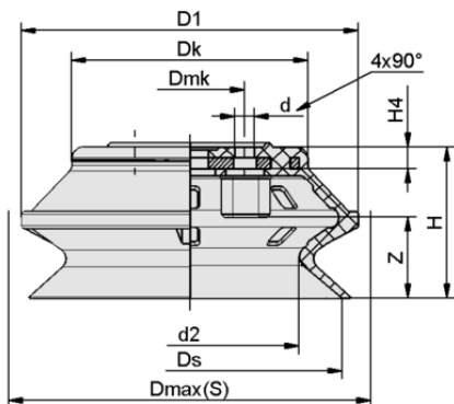
Конструктивные данные FGA 110 NBR-55 N010
