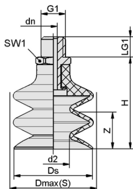
Конструктивные данные FSG 12 NK-45 M5-AG
