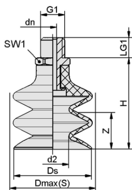
デザインデータ FSG 12 NBR-55 G1/8-AG
