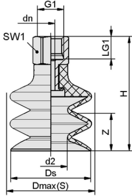
Tasarım verileri FSG 12 NBR-55 G1/8-IG
