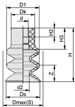
Données de construction FG 12 SI-55 N016
