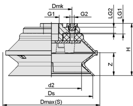
Datos de diseño FSGA 110 VU1-72 G1/2-IG ON
