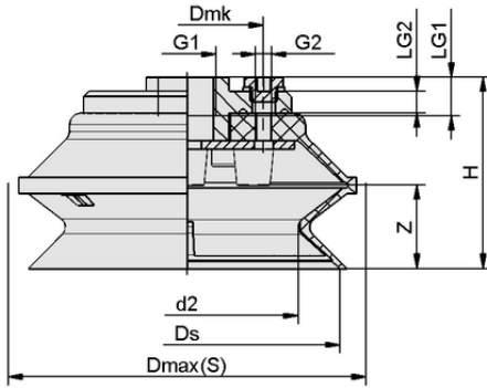
Tasarım verileri FSGA 110 VU1-72 G1/2-IG ON
