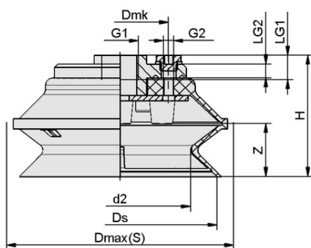
Конструктивные данные FSGA 110 VU1-72 G1/2-IG ON
