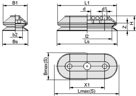
Tasarım verileri FGAO 140x65 VU1-72 N039
