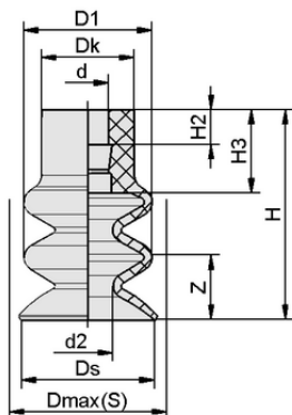
Datos de diseño FG 20 NK-45 N016
