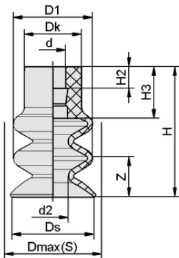
Datos de diseño FG 14 NK-45 N016
