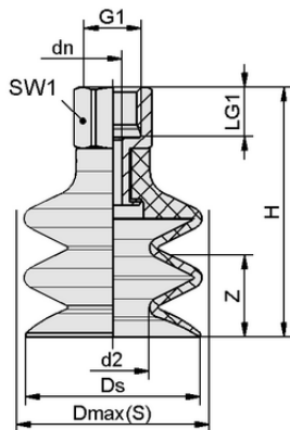
デザインデータ FSG 25 NK-45 G1/8-IG
