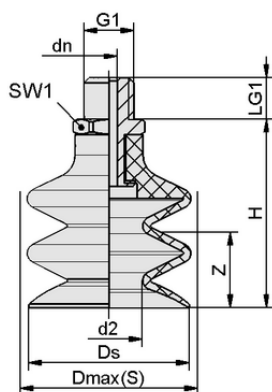
デザインデータ FSG 18 NK-45 M5-AG
