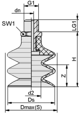
Tasarım verileri FSG 14 NK-45 M5-AG
