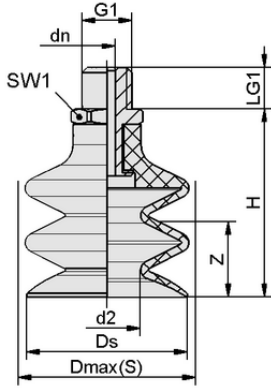
Tasarım verileri FSG 9 NK-45 M5-AG
