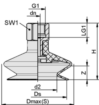
Données de construction FSGA 22 NK-45 G1/8-IG
