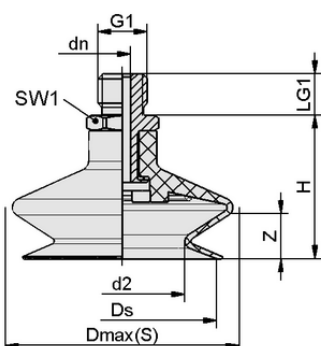
Конструктивные данные FSGA 22 NK-45 M5-AG
