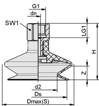
Конструктивные данные FSGA 16 NK-45 G1/8-IG
