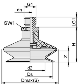
デザインデータ FSGA 20 NK-45 M5-AG
