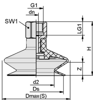
デザインデータ FSGA 20 SI-55 G1/8-IG
