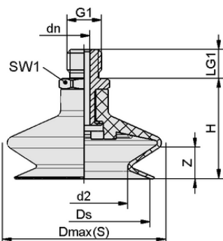
Datos de diseño FSGA 20 NBR-55 M5-AG
