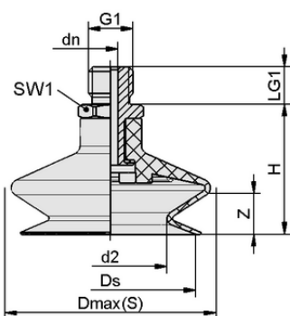
Конструктивные данные FSGA 14 NK-45 G1/8-AG
