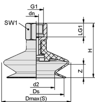
Données de construction FSGA 14 NK-45 G1/8-IG
