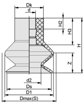
Datos de diseño FGA 20 NBR-55 N016
