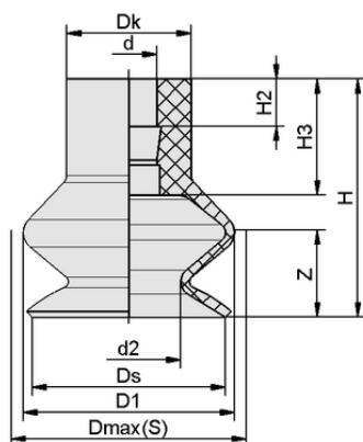
Конструктивные данные FGA 14 NK-45 N016
