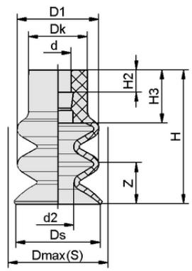
Données de construction FG 25 SI-55 N016
