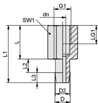
Конструктивные данные SA-NIP N017 M5-IG DN200
