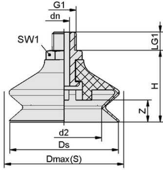
Tasarım verileri FSGA 40 VU1-72 G1/4-AG ON
