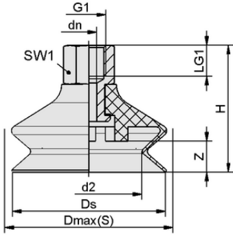
Tasarım verileri FSGA 60 VU1-72 G1/4-IG
