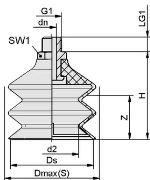
デザインデータ FSG 85 VU1-72 G1/4-AG
