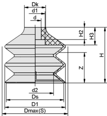
Datos de diseño FG 85 VU1-72 N015 ON
