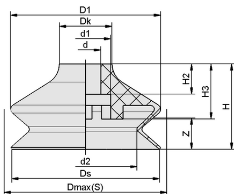
Конструктивные данные FGA 60 VU1-72 N014 ON
