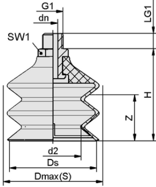
Tasarım verileri FSG 85 VU1-72 G1/4-AG ON
