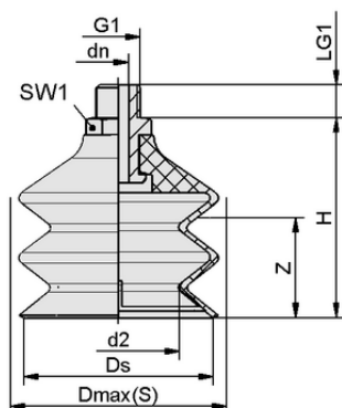
Конструктивные данные FSG 85 VU1-72 G1/4-AG ON
