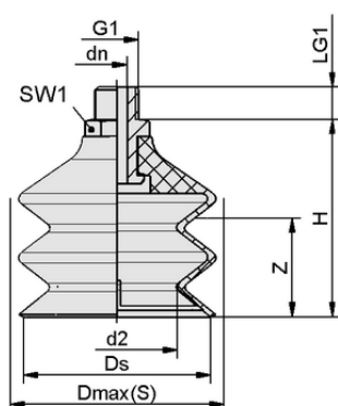
Конструктивные данные FSG 30 VU1-72 G1/4-AG
