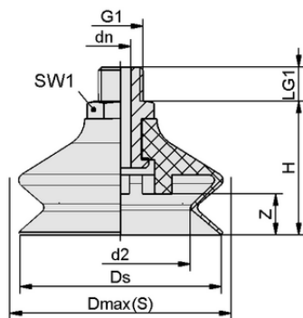
デザインデータ FSGA 30 VU1-72 G1/4-AG
