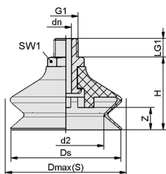
Конструктивные данные FSGA 30 VU1-72 G1/4-AG
