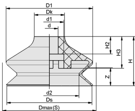
デザインデータ FGA 85 VU1-72 N015 ON
