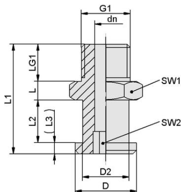
Конструктивные данные SA-NIP N013 G1/4-AG DN350
